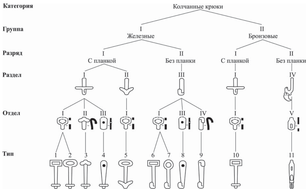
Рис. 1. Схема классификации колчаных крюков населения Алтая хуннско-сяньбийско-жужанского времени
